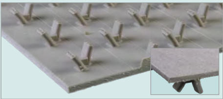
7 AGRU Sure Grip®-Betonschutzplatte PP grau kaschiert mit Polyestergewebe
